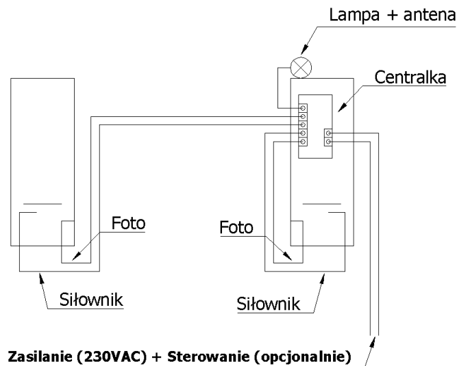
Rys. nr 3. Instalacja sterownika na słupku bramowym.
